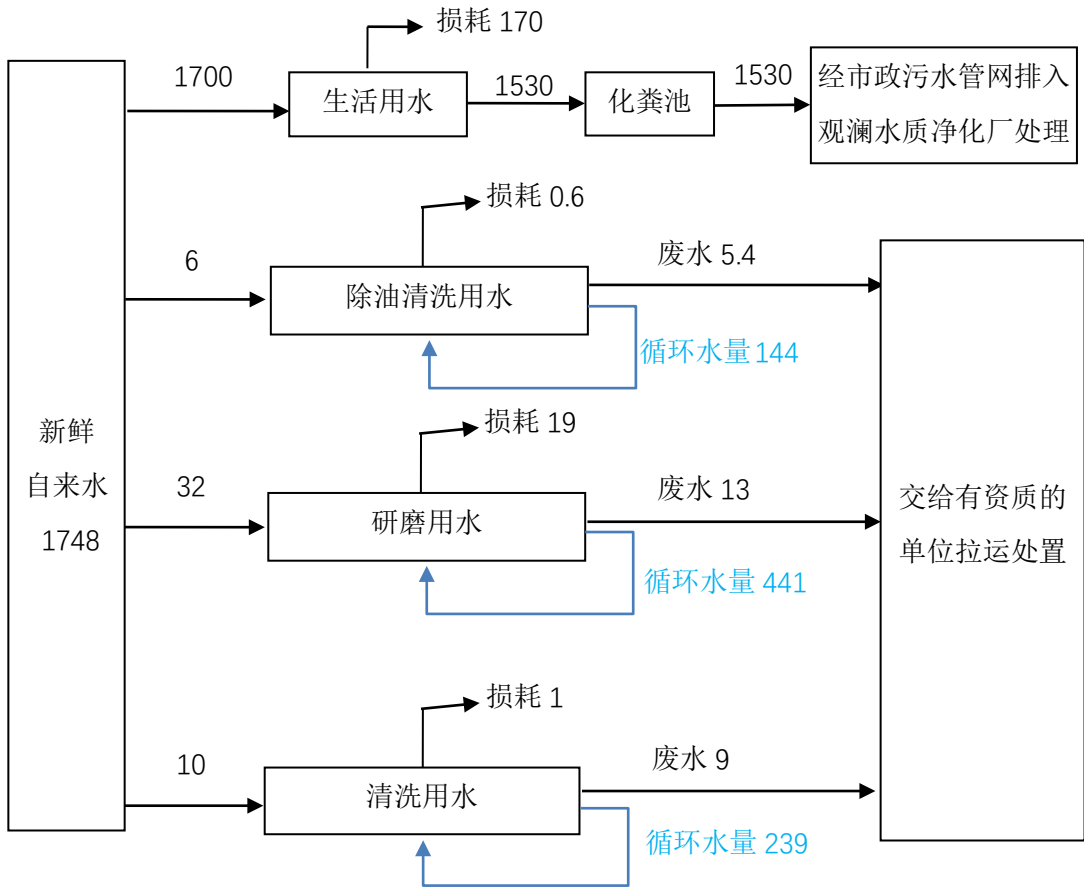
图 4-1 项目水平衡图 单位: t/a
