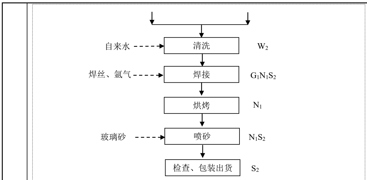
图 2-1 项目生产工艺流程图
