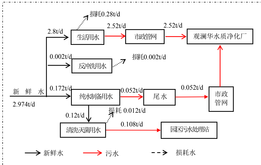
图 4-1 项目全厂用水平衡图
