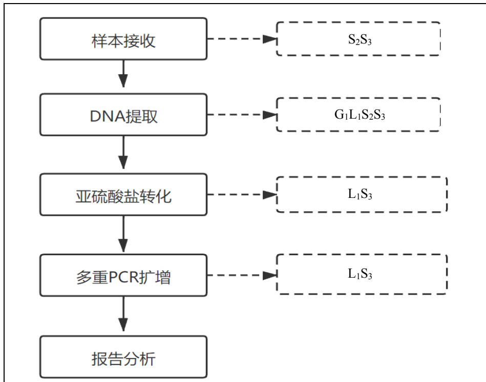
图 2-3 项目肿瘤早诊早筛研发工艺流程图
