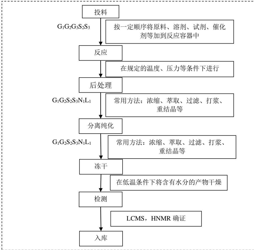
图 2-1 项目工艺流程图
